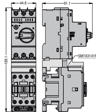
SM1R... mit Schützen BF09A...BF25A... und Anschluss SM1X3141R
