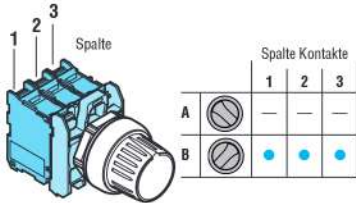
Wahlschalter mit Drehknopf mit 2 Positionen
