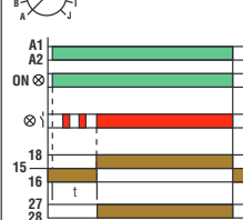
Verzögertes Ansprechen des Relais
