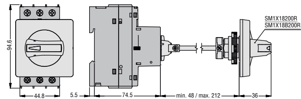
SM1R... mit abschließbarer Türverriegelung SM1X18200R oder SM1X18B200R
