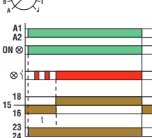
Verzögertes Ansprechen des Relais
