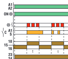
Zeitgesteuertes Ansprechen des Relais bei Schließen eines Kontakts
