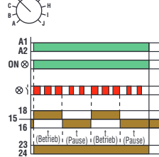
Blinken bei Betriebsbeginn
