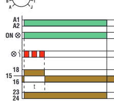
Verzögertes Abfallen des Relais
