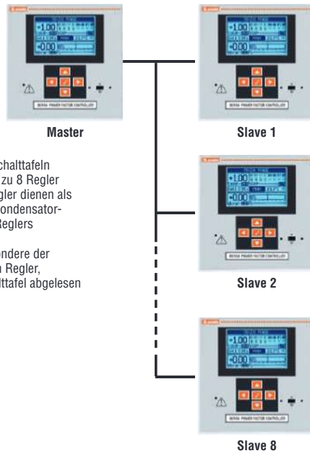
Kompensationssystem "Master-Slave" bei DCRG 8
