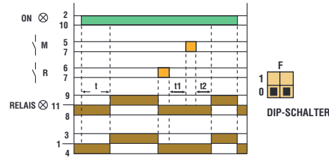
Verzögertes Ansprechen des Relais
