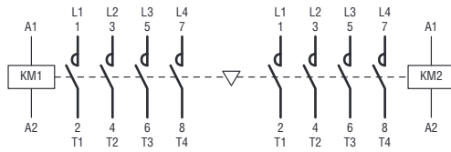
ZUSAMMENGEBAUTE UMSCHALTSCHÜTZE BGC09...
