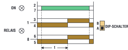
Verzögertes Ansprechen des Relais
