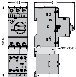
SM1R... mit Minischützen BG... und Anschluss SM1X3040R
