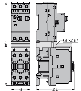
SM1P... mit Schützen BF26A...BF38A... und Anschluss SM1X3241P
