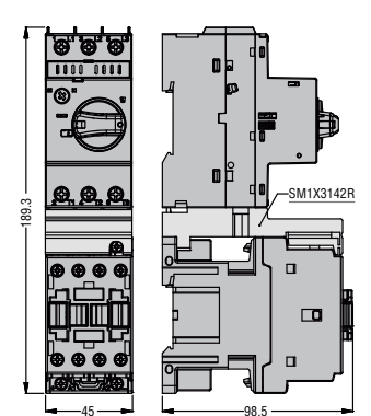
SM1R... mit Schützen BF09D...BF25D... BF09L...BF25L... und Anschluss SM1X3142R
