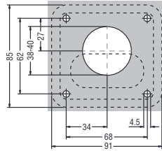
Einbauausschnitt
