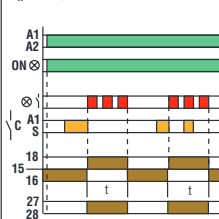
Zeitgesteuertes Ansprechen des Relais bei Öffnen eines Kontakts
