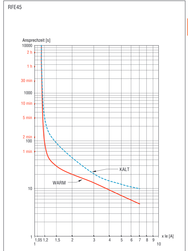
3-phasiger symmetrischer Betrieb, Klasse 30
