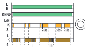
Zeitgesteuerte Einschaltung mit Ausschaltvorwarnung + Einschaltung für Treppenreinigung
