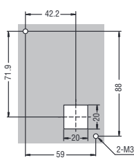
Einbauausschnitt
