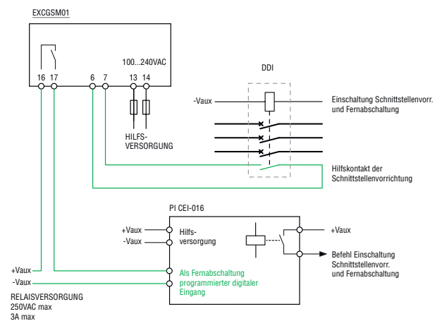
Anschlussplan Modem EXCGSM01 mit weiteren Spannungs- und Frequenzwächtern mit zu versorgendem Eingang für Fernabschaltung
