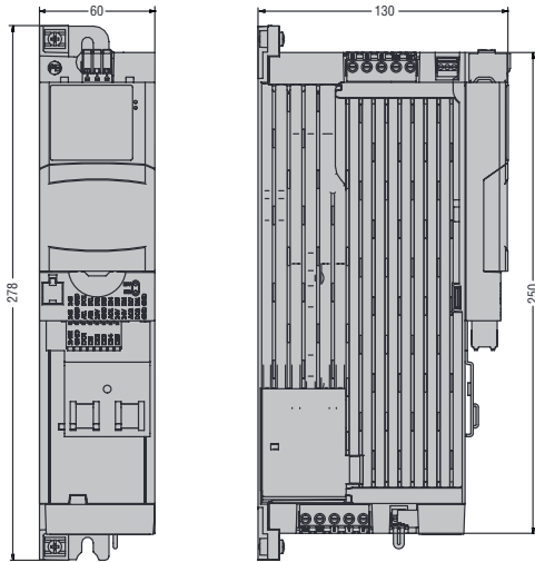
VLB30015A480 - VLB30022A480 - VLB30040A480
