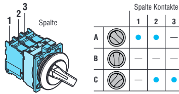
Wahlschalter mit Hebel mit 3 Positionen
