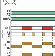
Schrittrelais bei Schließen des Kontakts
