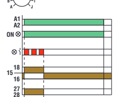
Verzögertes Abfallen des Relais
