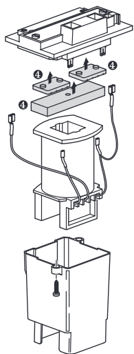
Spule komplett
