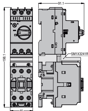
SM1R... mit Schützen BF26A...BF38A... und Anschluss SM1X3241R
