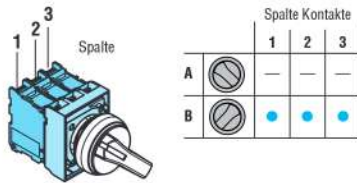
Wahlschalter mit Hebel mit 2 Positionen
