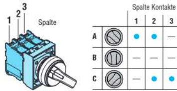
Wahlschalter mit Hebel mit 3 Positionen
