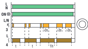
Zeitgesteuerte Einschaltung + Einschaltung für Treppenreinigung
