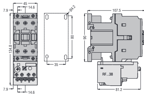
BF26... - BF32... - BF38... D und L 3-polig mit Überstromrelais RF...38
