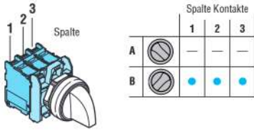
Wahlschalter mit Hebel mit 2 Positionen
