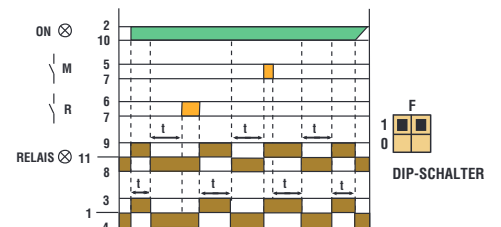
Blinken bei Betriebsbeginn
