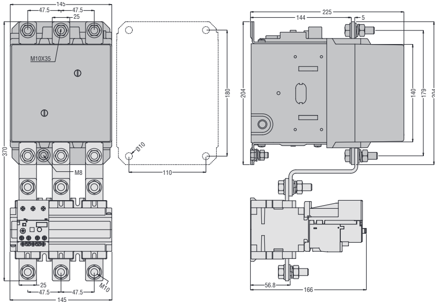
B250 - B310 - B400 3-polig mit Überstromrelais RF...420
