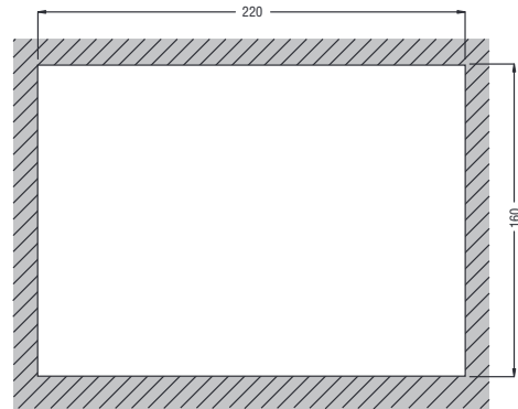
Einbauausschnitt
