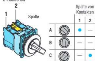
Betätigung der Kontakte, Wahlschalter mit 3 Positionen
