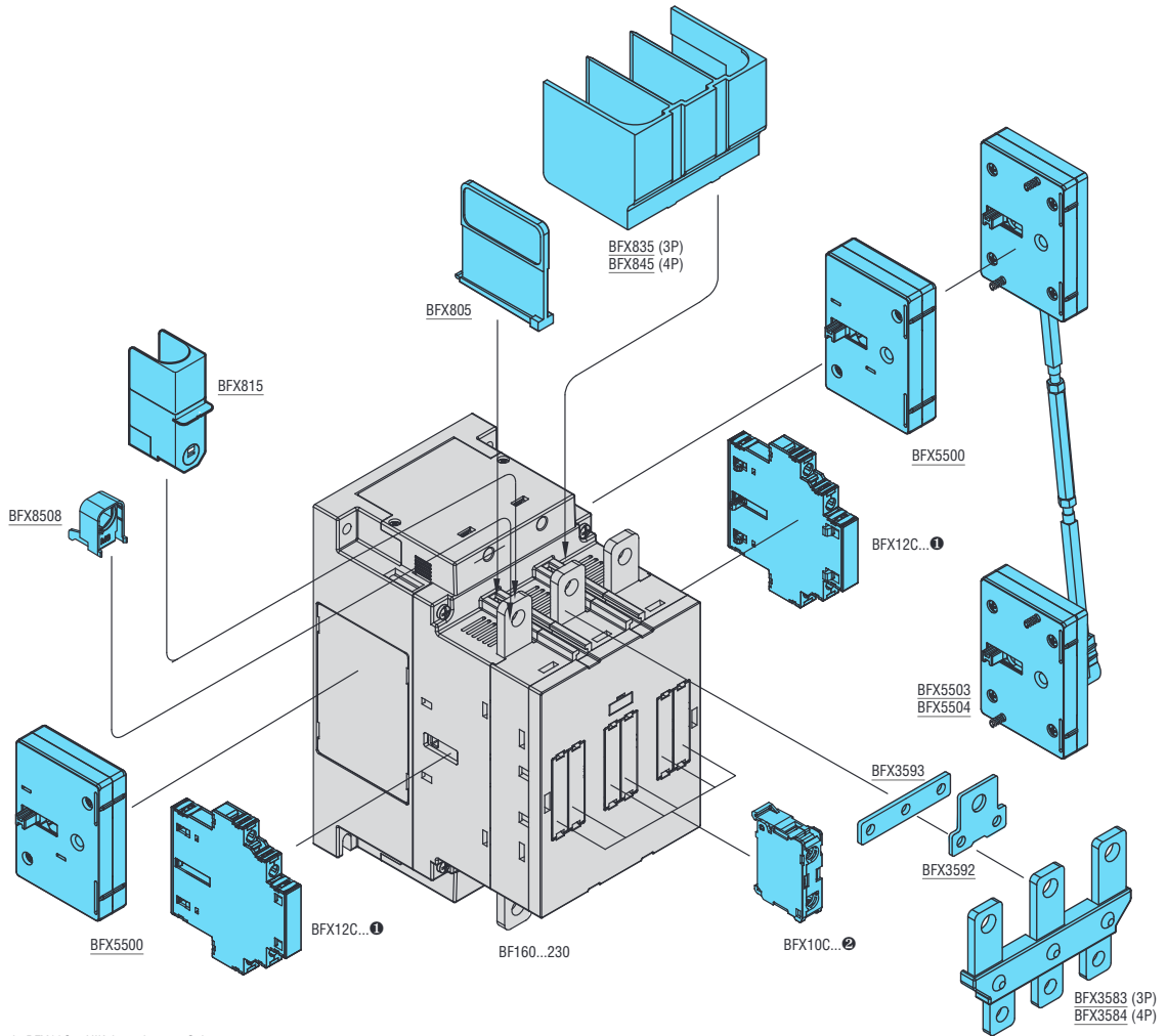
Anbaumöglichkeiten des Zubehörs für Schütze BF160...BF230
