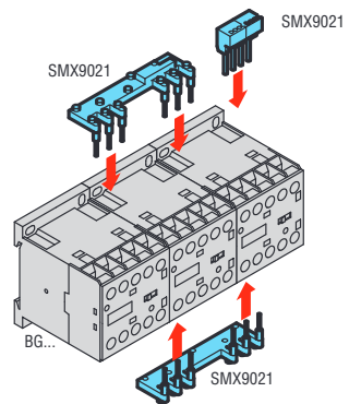
Anschlüsse für Stern-Dreieck-Starter
