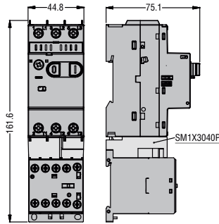
SM1P... mit Minischützen BG... und Anschluss SM1X3040P
