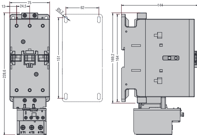
BF9500A... - BF11500A... - BF15000A... 3-polig mit Überstromrelais RF110
