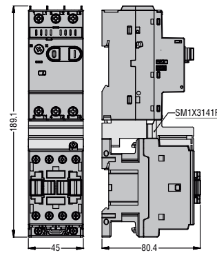
SM1P... mit Schützen BF09A...BF25A... und Anschluss SM1X3141P
