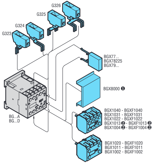
Anbaumöglichkeiten: Einbaulage auf Minischützen BG...A und BG...D
