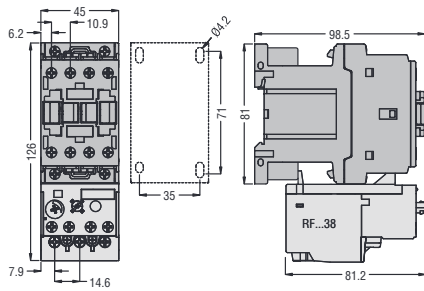
BF00...D und BF00...L BF09... - BF12... - BF18... - BF25...D und L 3-polig mit Überstromrelais RF...38
