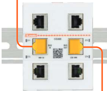
EXS4000 Strommessmodul mit 4 Eingängen für elektronische Stromwandler RJ45
