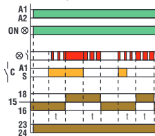
Verzögertes Ansprechen des Relais bei Schließen eines Kontakts und verzögertes Abfallen bei Öffnen
