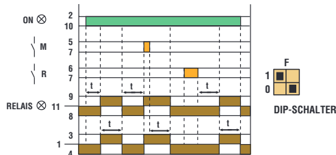
Blinken bei Pausenbeginn
