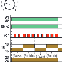
Blinken bei Pausenbeginn
