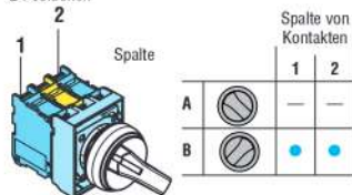
Betätigung der Kontakte, Wahlschalter mit 3 Positionen
