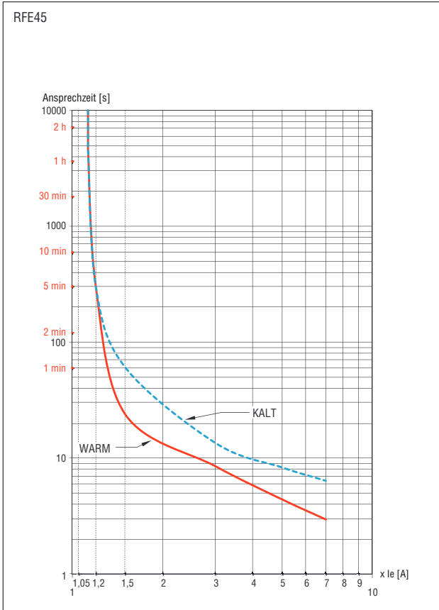
3-phasiger symmetrischer Betrieb, Klasse 20
