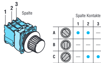
Wahlschalter mit Drehknopf mit 3 Positionen
