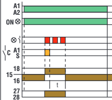
Ansprechen des Relais bei Schließen eines Kontakts und verzögertes Abfallen bei Öffnen
