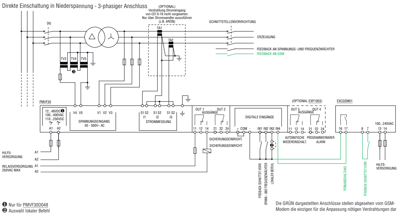
Anschlussplan Modem EXCGSM01 mit weiteren Spannungs- und Frequenzwächtern mit selbstversorgtem Eingang für Fernabschaltung
