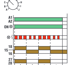
Blinken bei Betriebsbeginn
