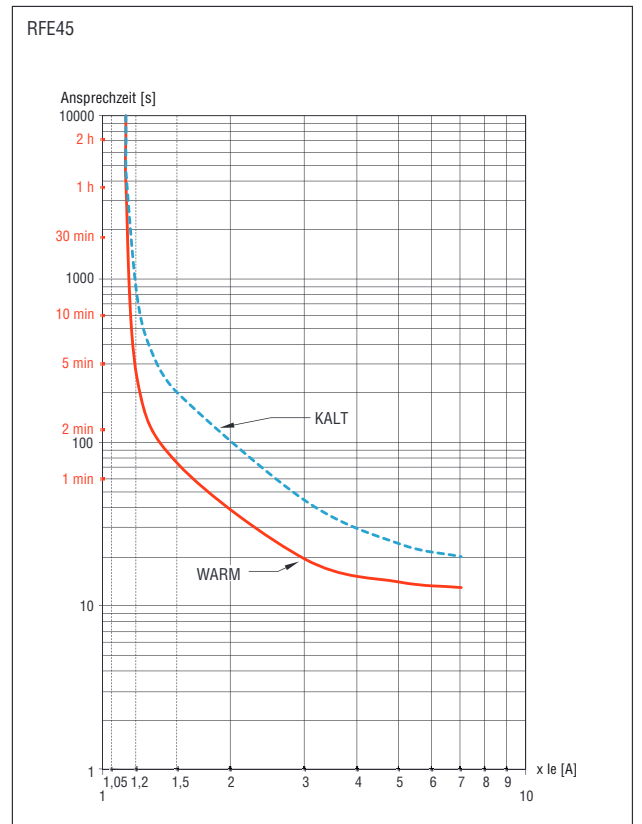
3-phasiger symmetrischer Betrieb, Klasse 30
