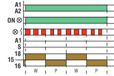
Blinken bei Betriebsbeginn
