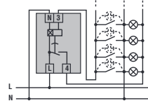
Anschluss mit 3 Drähten
