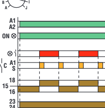
Schrittrelais bei Schließen des Kontakts
