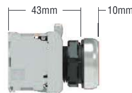
Aus Kunststoff, verchromt Ø22mm
