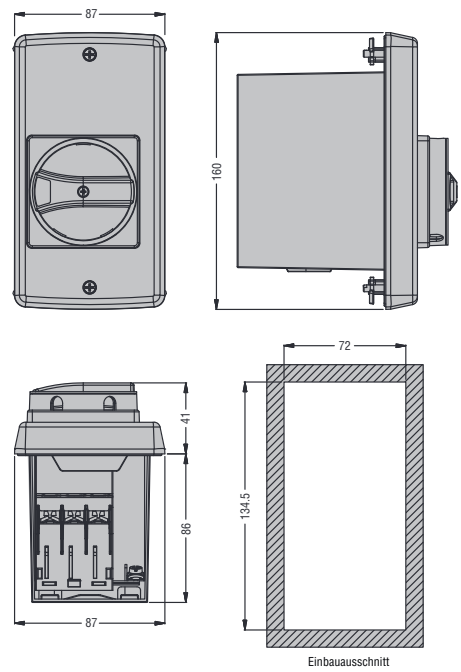
Gehäuse SM1Z1720R und SM1Z1725R
