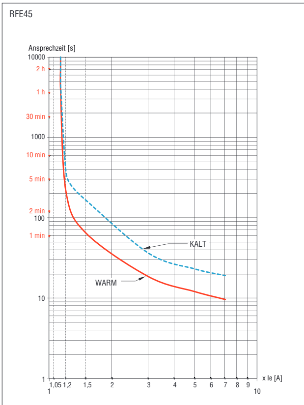
3-phasiger symmetrischer Betrieb, Klasse 20
