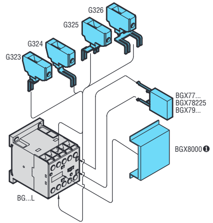
Anbaumöglichkeiten: Einbaulage auf Minischützen BG...L
