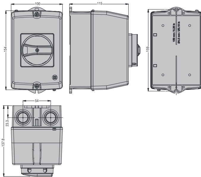
Gehäuse SM1Z1715R und SM1Z1710R
