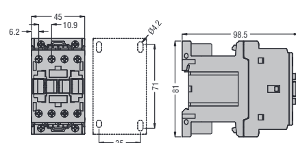
BF00...D und BF00...L BF09T... - BF18T... D und L 4-polig
